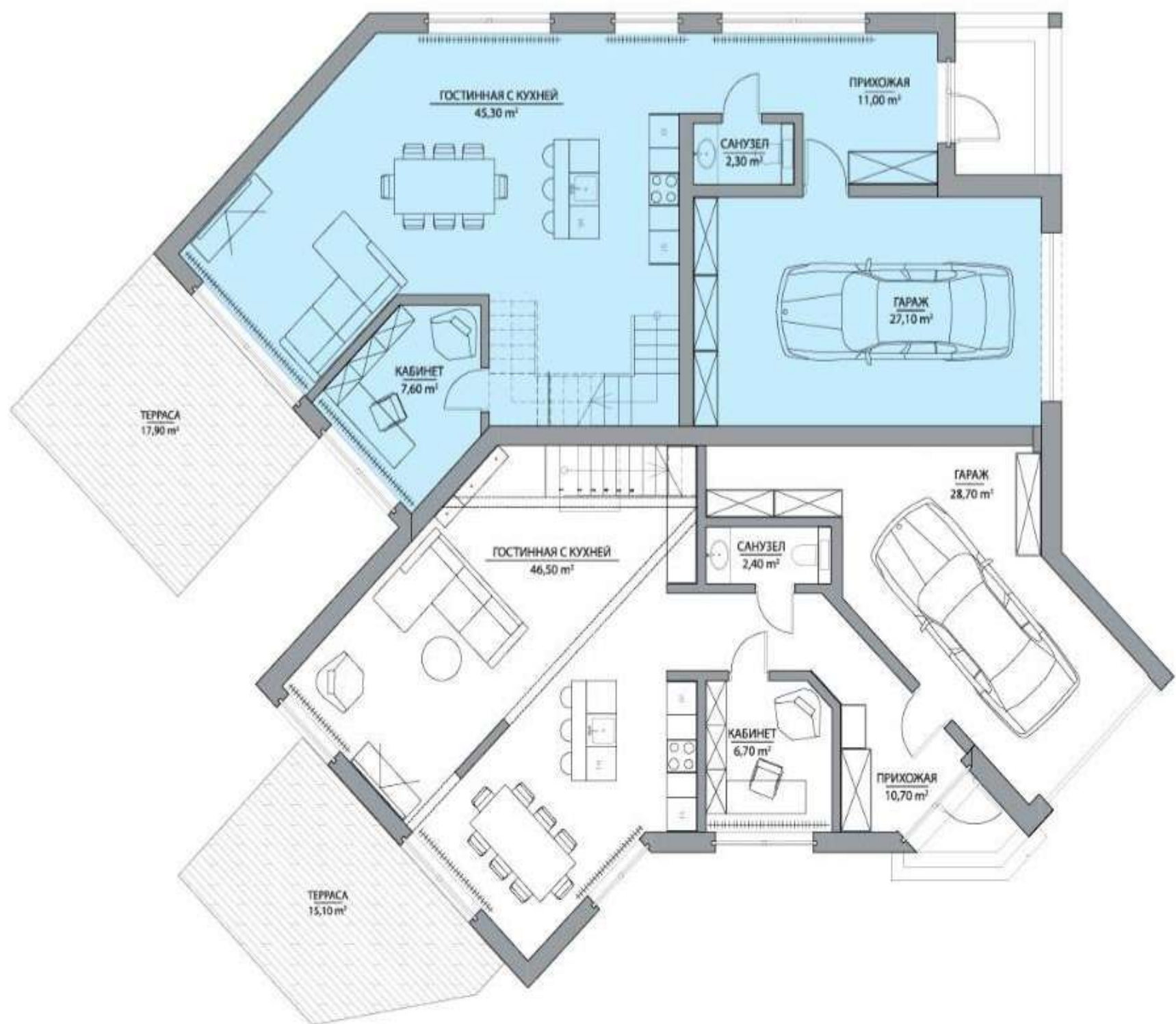
ПЛАН 1 ЭТАЖА
