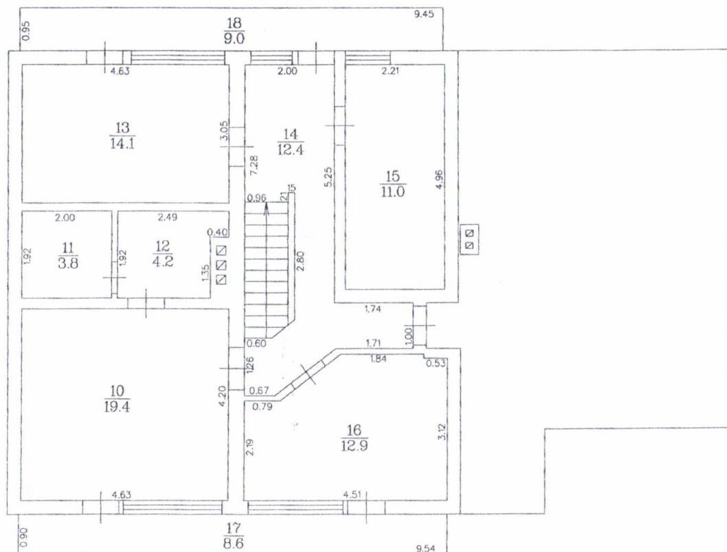
2. stāva plāns
