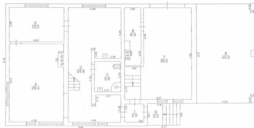
1. stāva plāns
